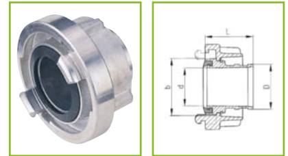
mit Einbindestutzen für Druckbetrieb 1001 (DS) und Saugbetrieb
