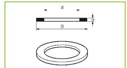
① Gewindedichtung flach
